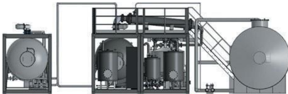
Рис. 3. Мобильный комплекс по переработке отработанных масел
